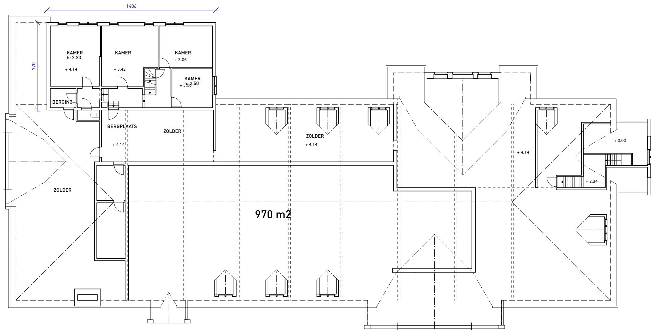
VERDIEPING 1
